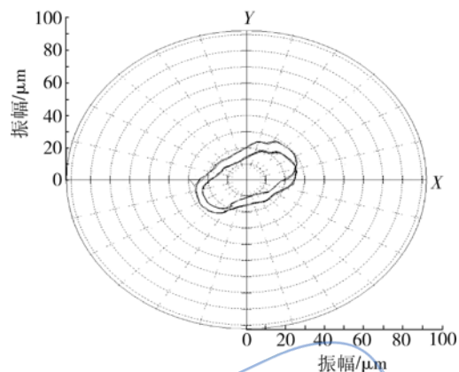
(a) 试验1 (转速为14769 r/min)
