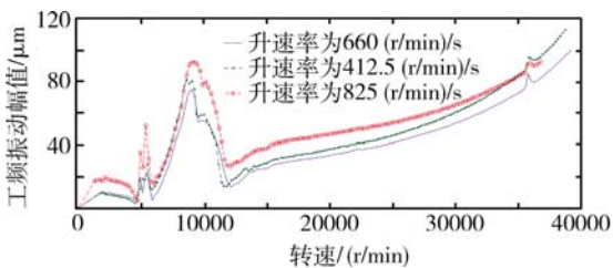
图 6 不同升速率下转速-幅值曲线(涡轮端)
