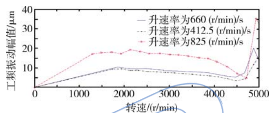
图 7 转速-幅值曲线(0~5 000 r/min)局部放大
