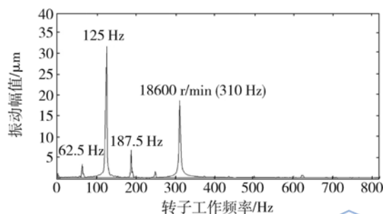
(a) 试验1 (转速为18600 r/min时的频谱图)
